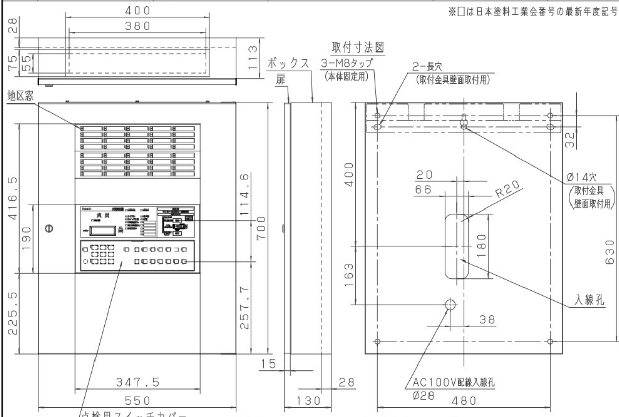
取付寸法図 (取付金具) ダルマ穴寸法図 (本体) 取付金具
