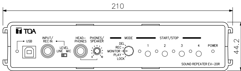
正面図
