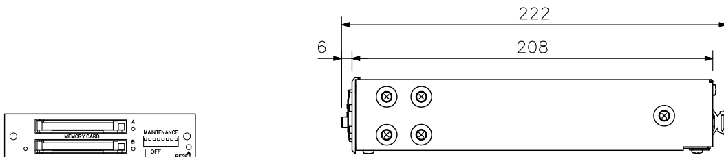
フロントカバーを外した図
